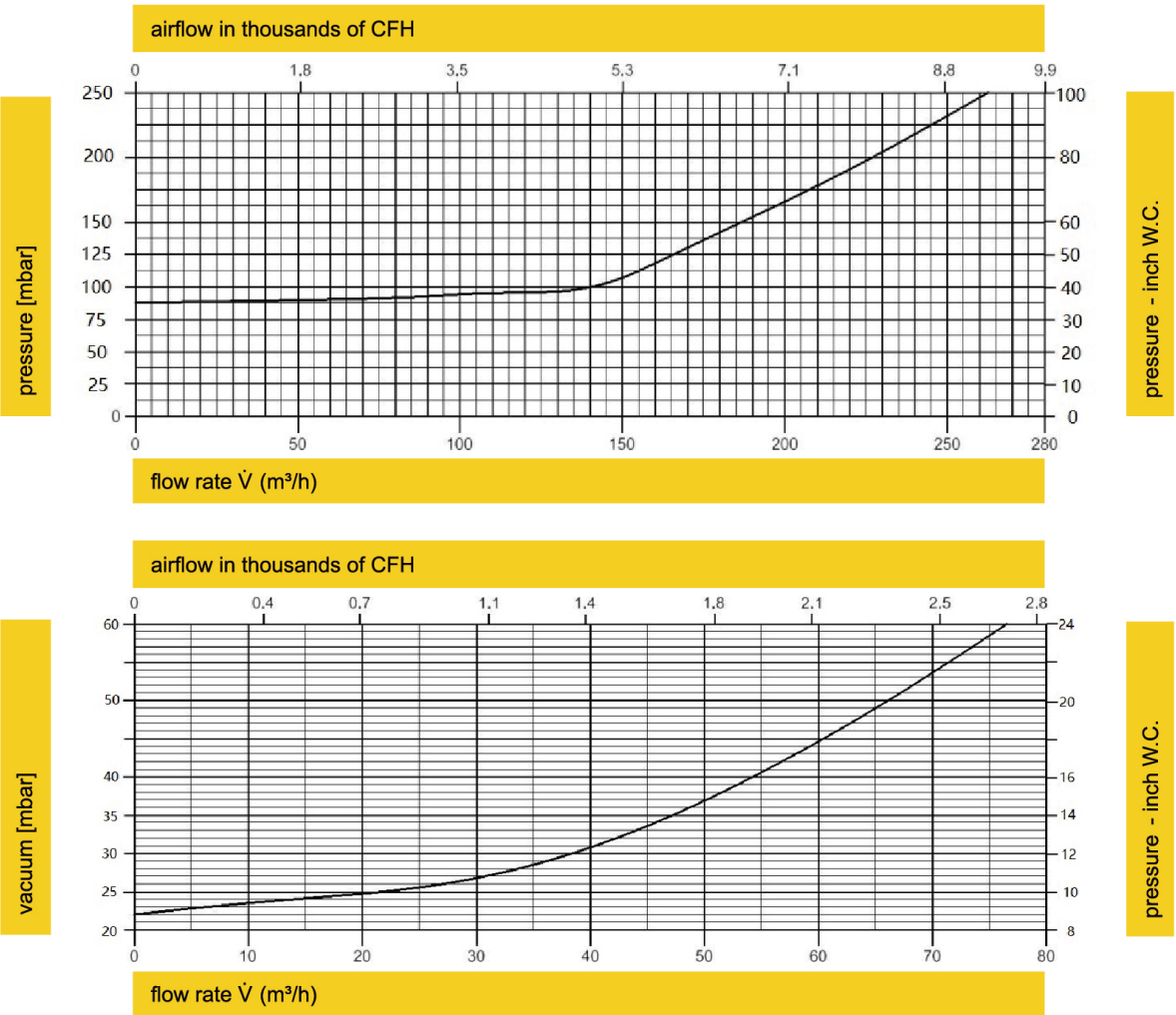
流量图 Flow Capacity Chart
